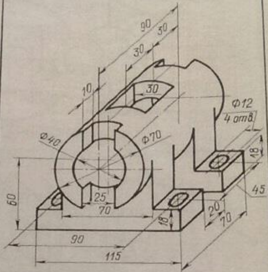
Корпус
