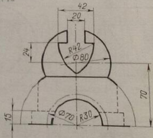
Корпус
