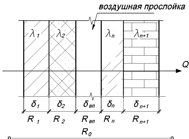
Рис.2. Общее сопротивление теплопередаче ограждения
