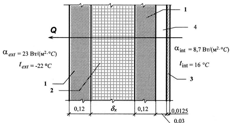
Рис.1. Расчетная схема к теплотехническому расчету
