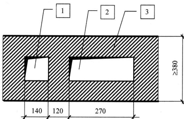
Рис. 1. Вентиляционные каналы в кирпичной стене 1 – вентиляционный канал сечением 140×140 мм; 2 – вентиляционный канал сечением 140×270 мм; 3 – кирпичная стена
