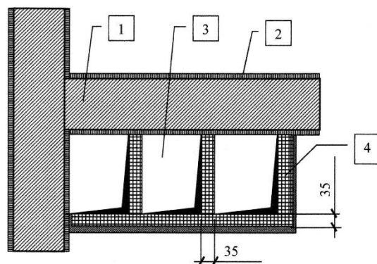
Рис. 2. Приставные вентиляционные каналы 1 – внутренняя стена; 2 – штукатурка; 3 – вентиляционный канал; 4 – шлакогипсовые плиты.
