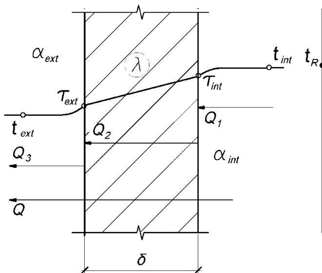
Рис. 1. Расчетная схема
