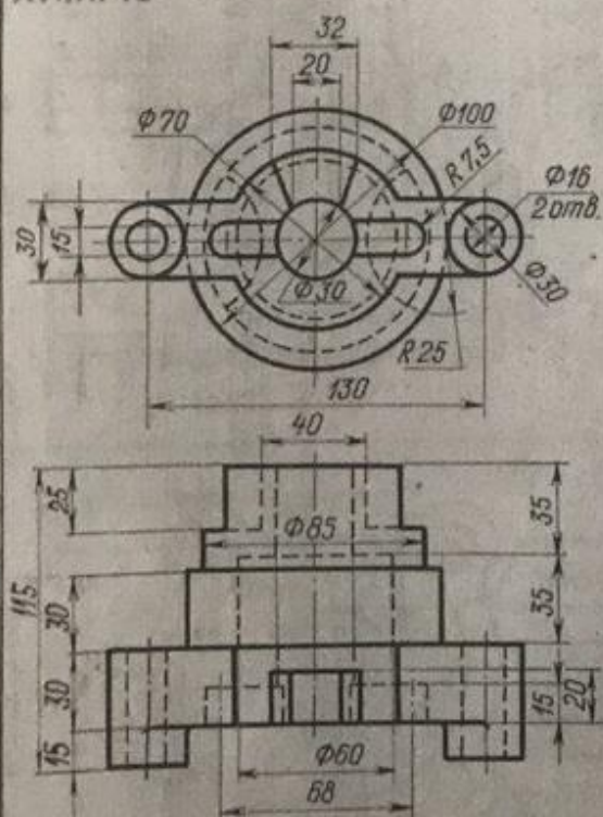
Траверса
