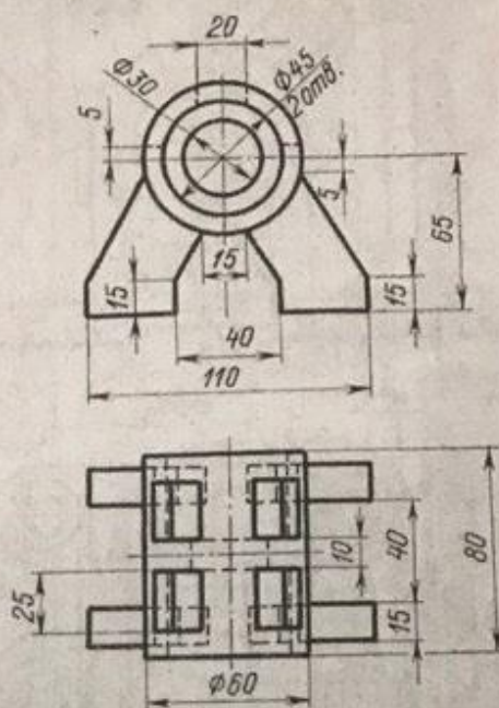
Стійка
