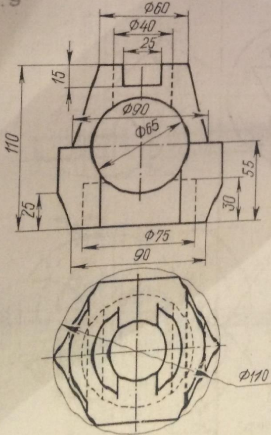
Опора
