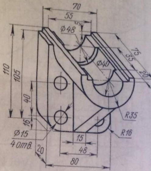
Кронштейн
