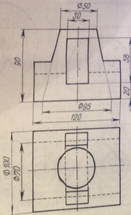
Кронштейн
