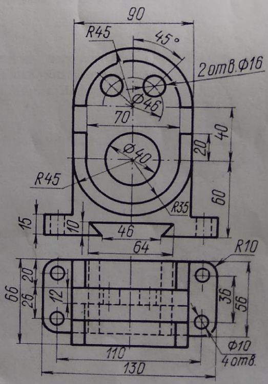
Стойка
