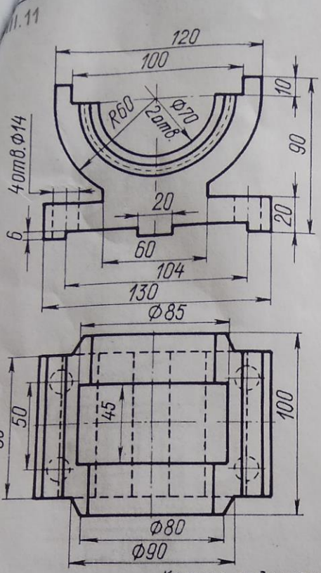
Корпус подшипника
