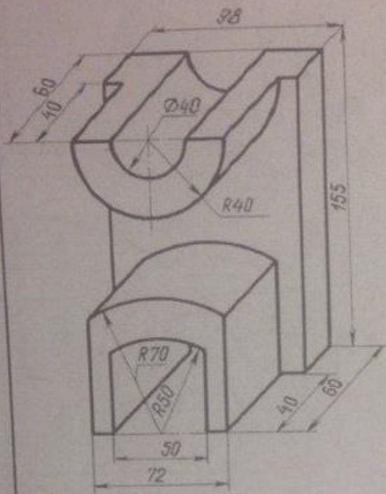
Опора
