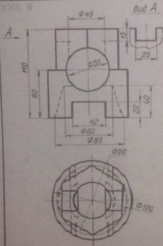
Опора
