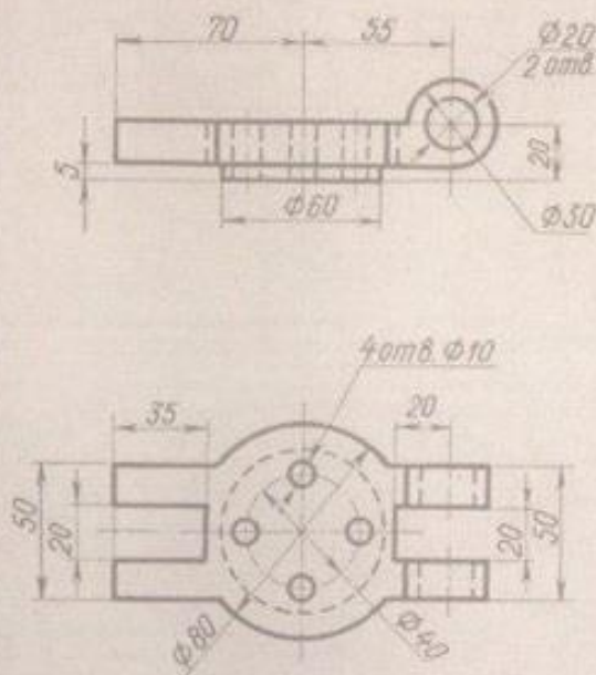
Крышка
