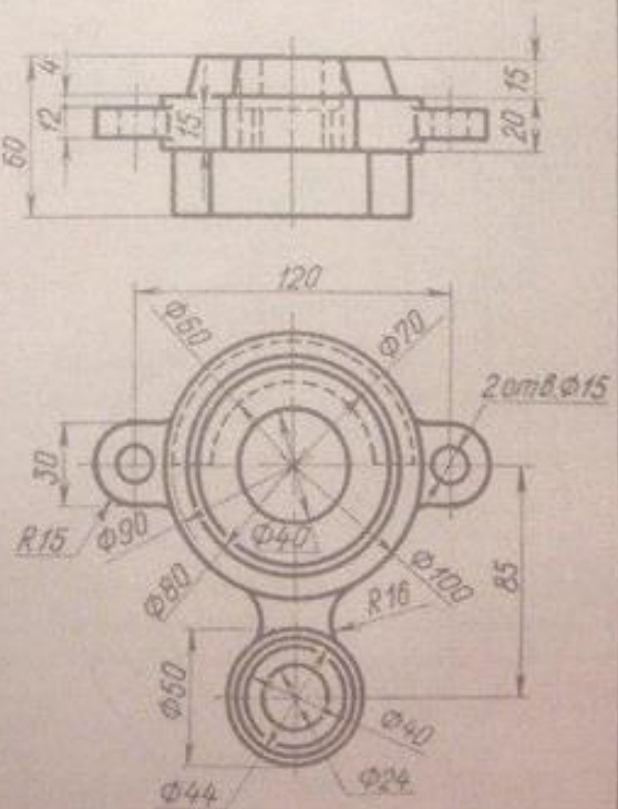
Серьга
