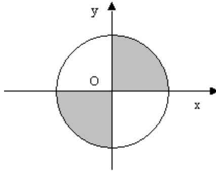
Рис.3.7. Заданная область плоскости
