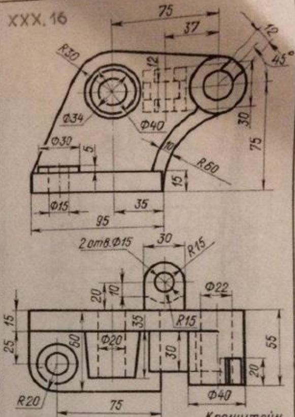
Кронштейн
