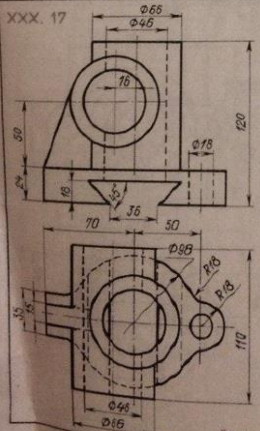
Корпус
