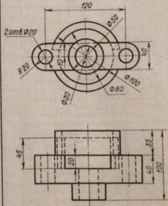
Щиток
