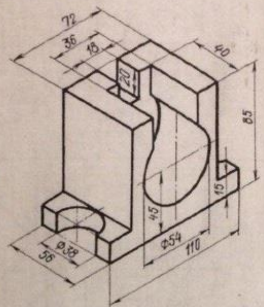
Опора
