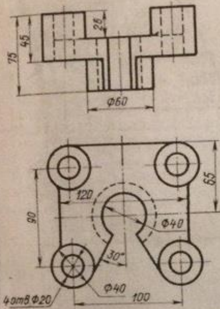
Прижим
