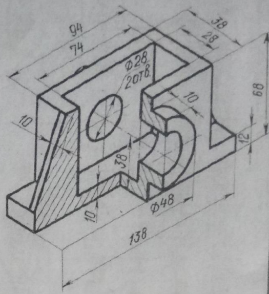
Корпус
