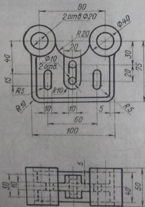
Подвеска
