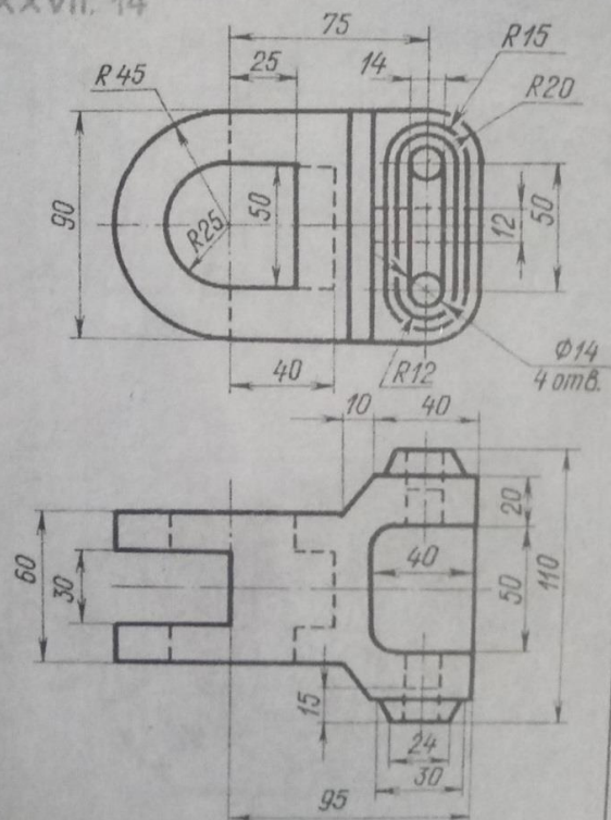
Вилка
