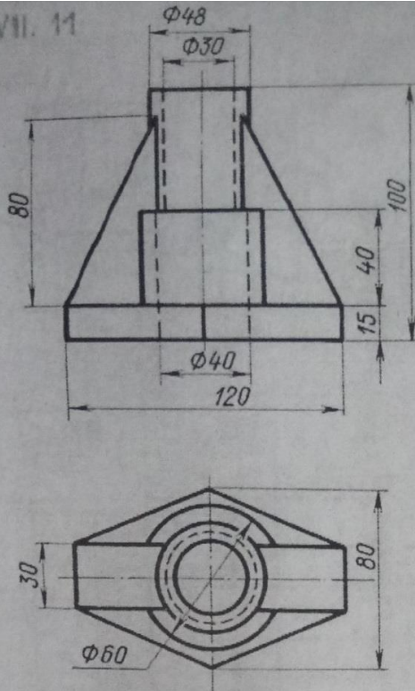
Стойка
