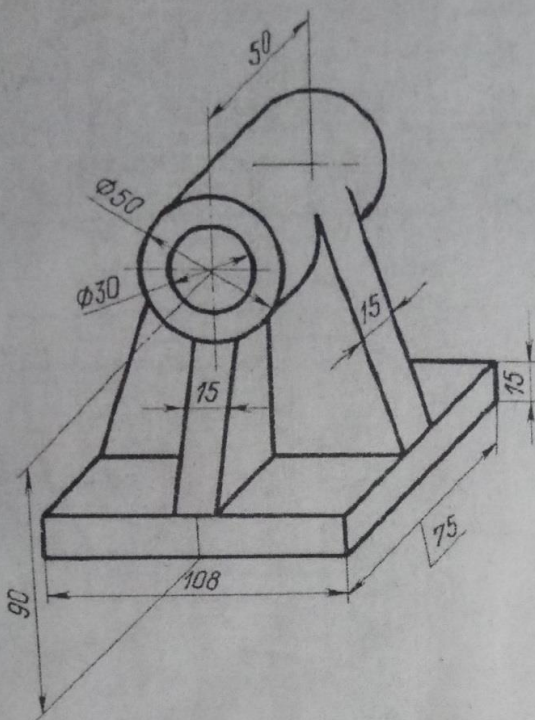
Подшипник
