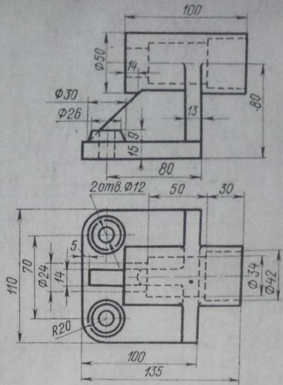
Подшипник
