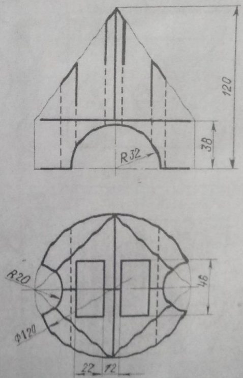
Корпус
