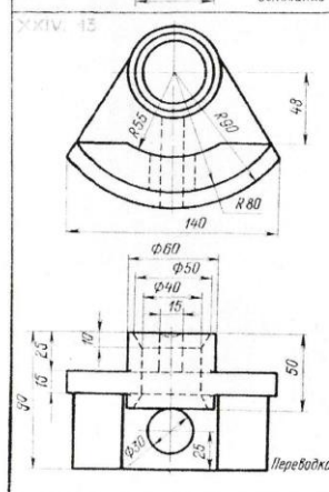
Основа
