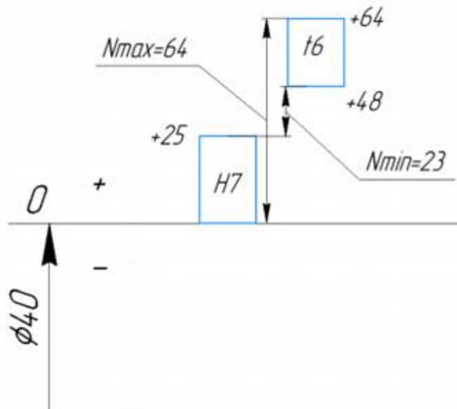
Рисунок -2 Схема расположения интервалов допуска посадки с натягом
