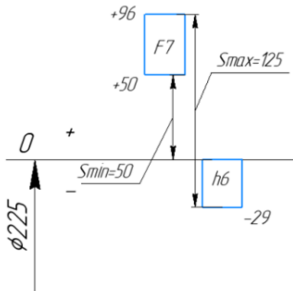
Рисунок -1 Схема расположения интервалов допуска посадки с зазором
