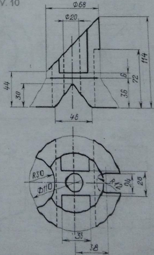
Подпятник
