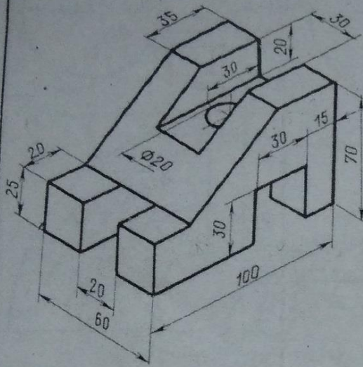
Опора
