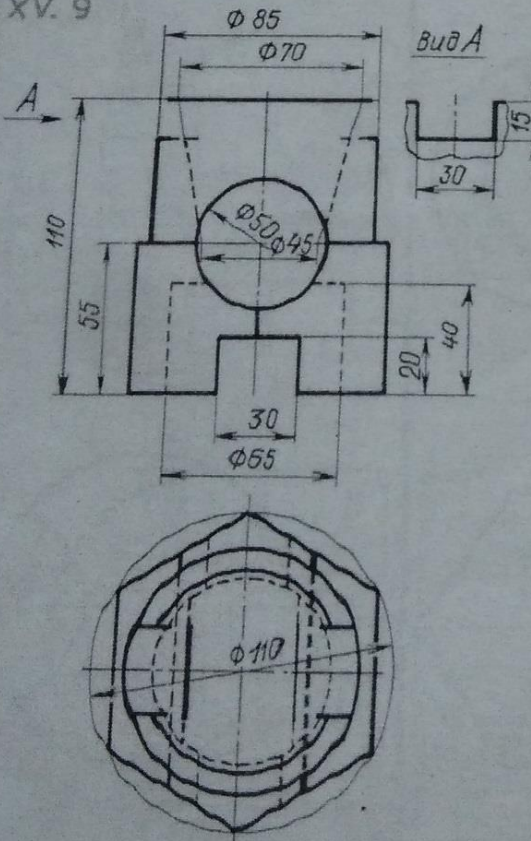
Опора
