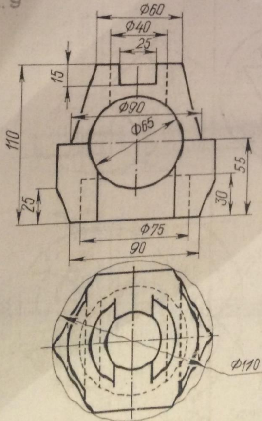
Опора
