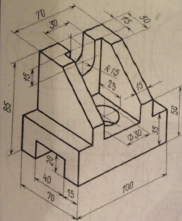
Опора
