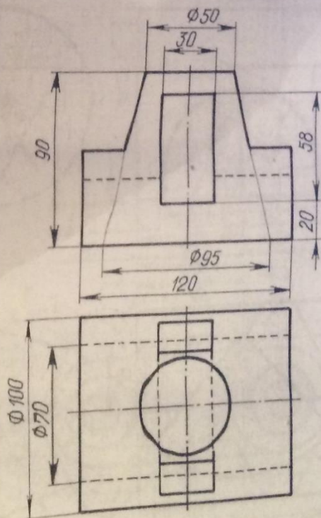
Кронштейн
