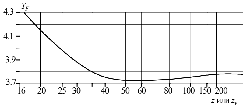
Рис. 4.2. Значение коэффициента формы зуба Y_F при коэффициенте смещения X=0 в зависимости от числа зубьев z (для косозубых и конических - эквивалентное число зубьев z_v )
