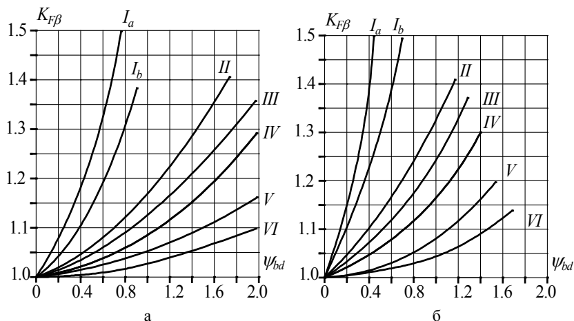
Рис. 5.1. Значения коэффициента K_{F\beta} для цилиндрических передач в одноступенчатом редукторе находится по графику V : а – значение коэффициента при HB_2 \leq 350 , б - значение коэффициента при HB_1 > 350 и HB_2 > 350 ;
