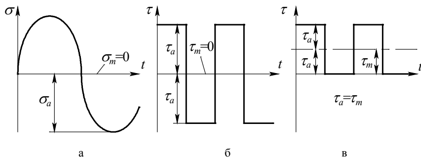
Рис. 6.1. Характер изменения величины напряжений в поперечном сечении вала: а – нормальных; б – касательных при реверсивной работе; в – касательных при не реверсивной работе.
